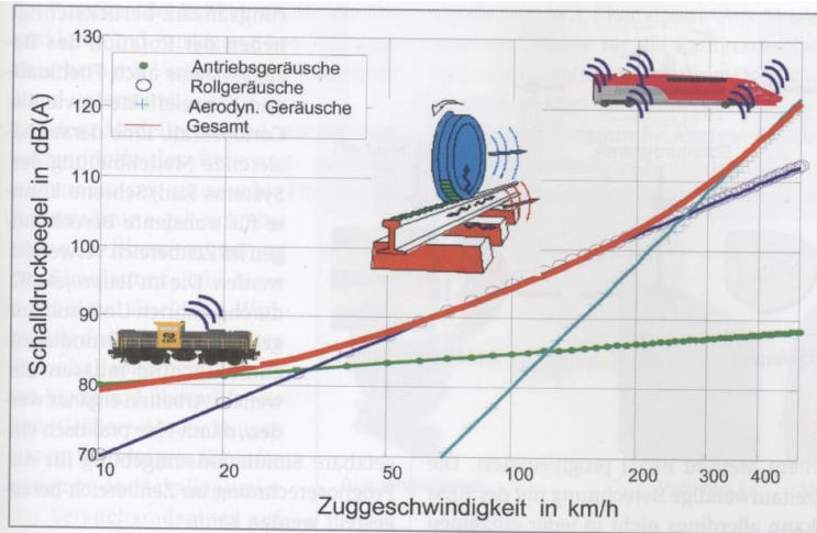
Bild 1: Schalldruckpegel von Schienenfahrzeugen in Abhängigkeit ihrer Fahrgeschwindigkeit
