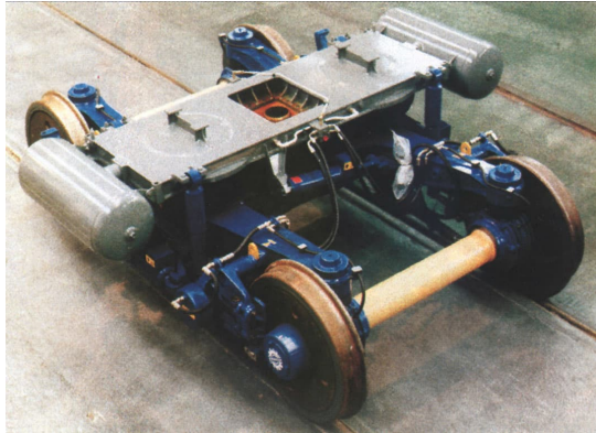
Leichtbaudrehgestell B 5003 (3,3t) der Firma Bombardier-Talbot
