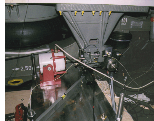
Versuchsanordnung
