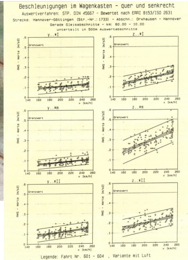
RMS- Werte des Drehgestells B 5003 unter Nahverkehrswagen Horizontal- quer und vertikal
