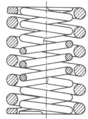
Stahl-Schraubenfeder
