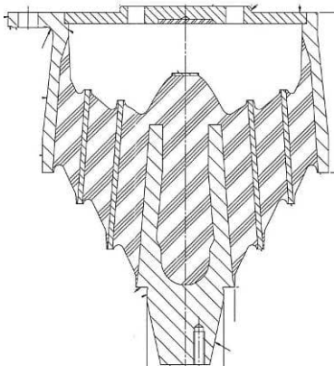
Gummi-Konusfeder
