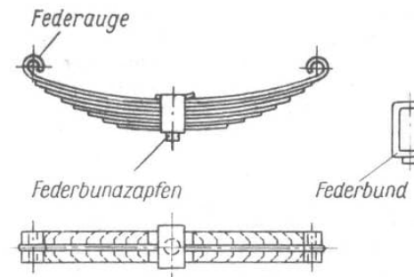
Blattfeder
